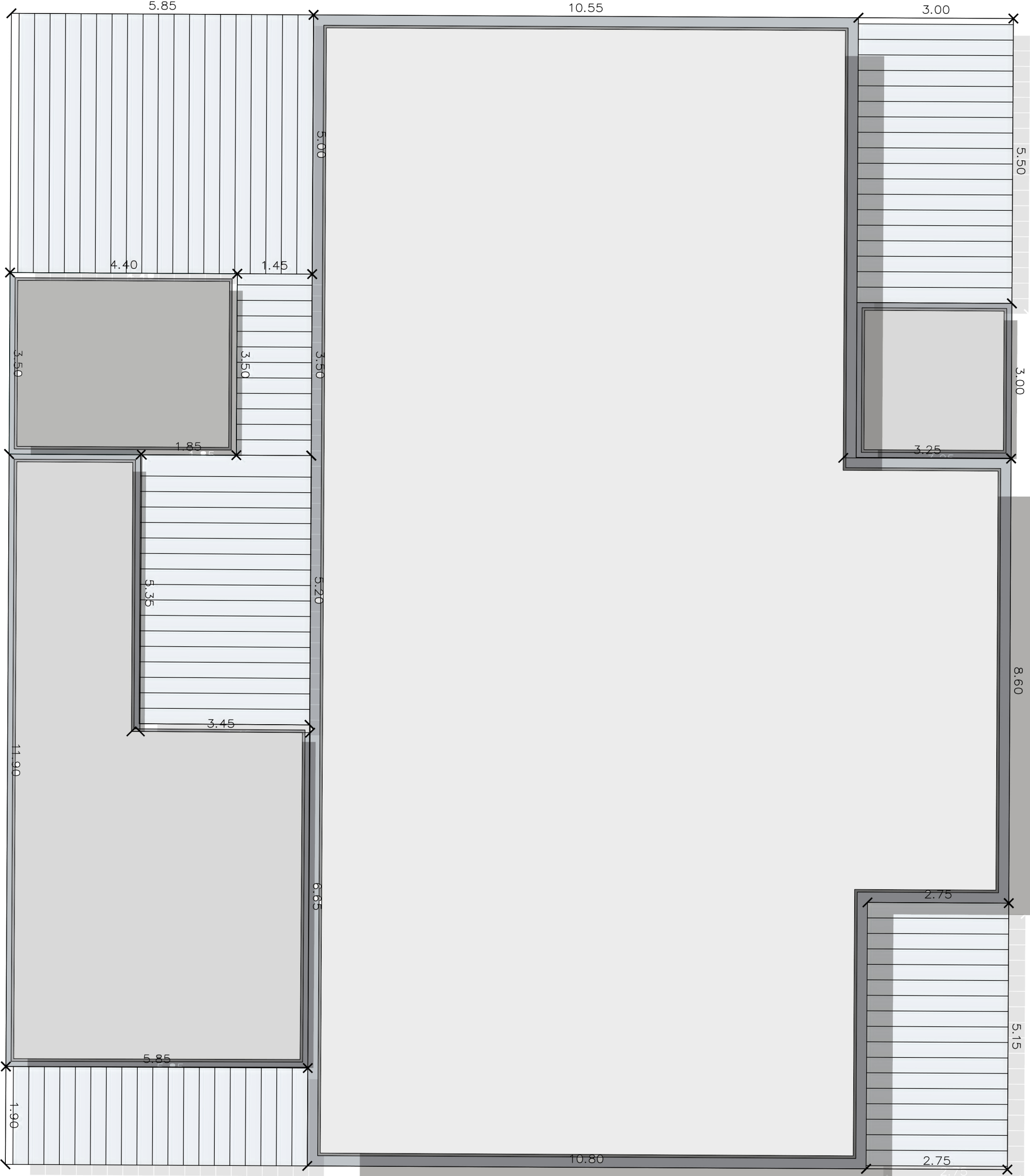
PLAN INVELITOARE 1/50
